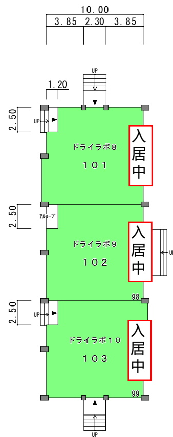
1階平面図 296㎡
