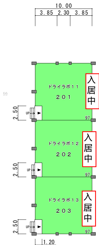
2階平面図 291㎡
